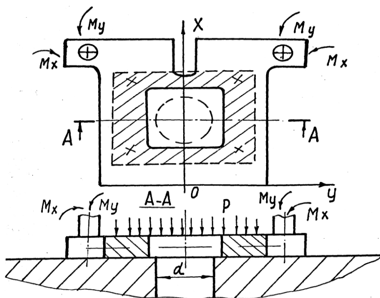
Рис.1. Схема нагружения нижней плиты
