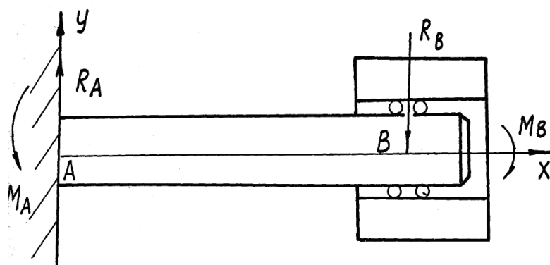
Рис. 2. Схема нагружения направляющей колонки
